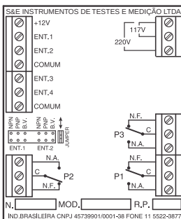
UNIDADE ELETRÔNICA CAIXA 96 x 96 mm
